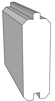
B3 (1x) 38x121x195mm
